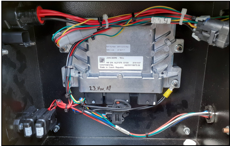
Schaltschrank komplett für FSW IsoBus
