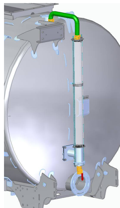
Variante: Pumpfasswagen / Rechts
