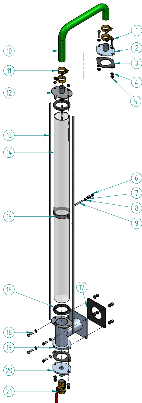
Variante: Vakuumfasswagen / Links
